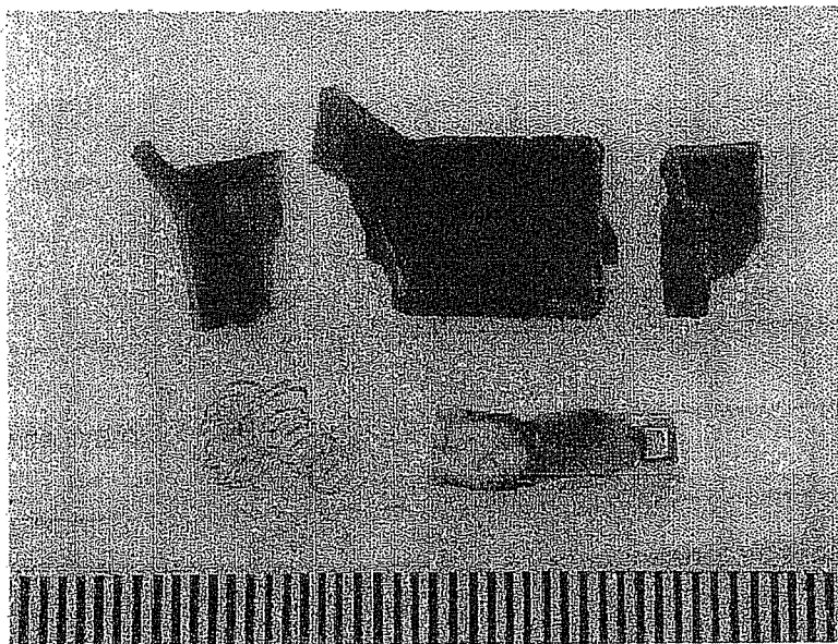
שרידי פלסטיק, קפיץ, ומגוע חשמלי שנראה ומקורם במפסק חשמלי כלשהו
